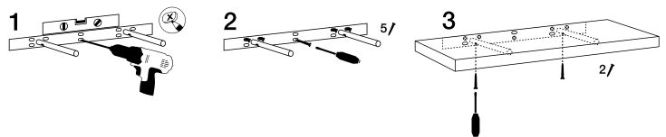
Tornillos de fijación a pared no incluidos. Vis de fixation au mur pas inclus. Fixing screw wall not included.
